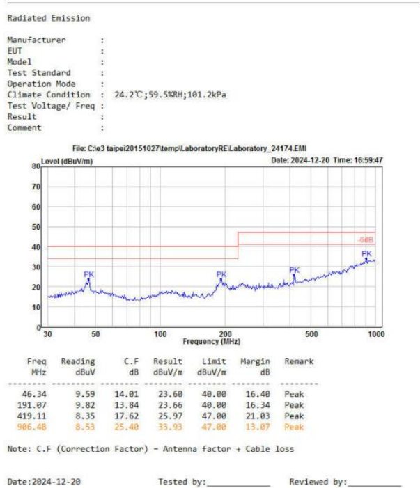
图 5-6 辐射测试水平方向
